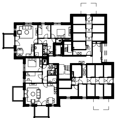
PLATTEGROND BOUWNUMMER. 1 Gebruiksoppervlakte 70.0m 2 Begane grond (Peil = 0)
